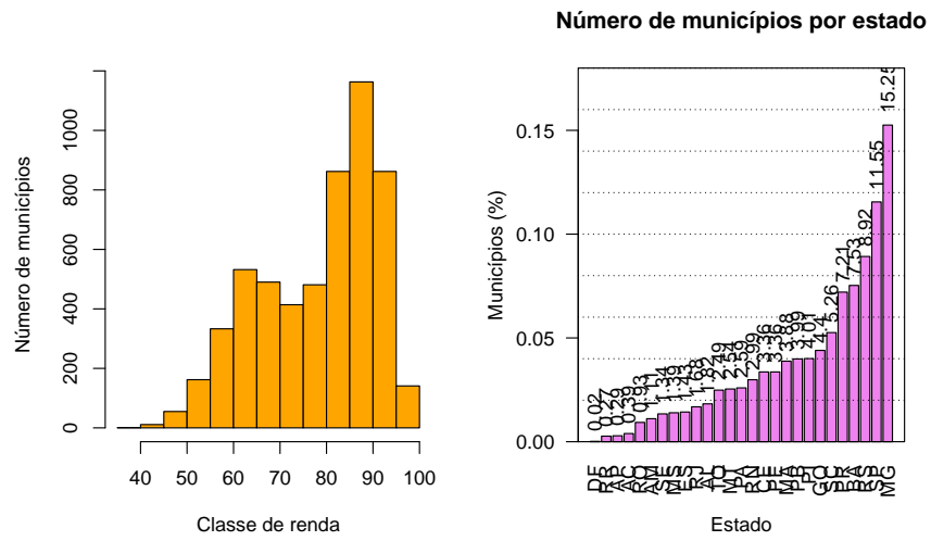
Figura 2: Gráfico de barras do número de municípios por estado.
