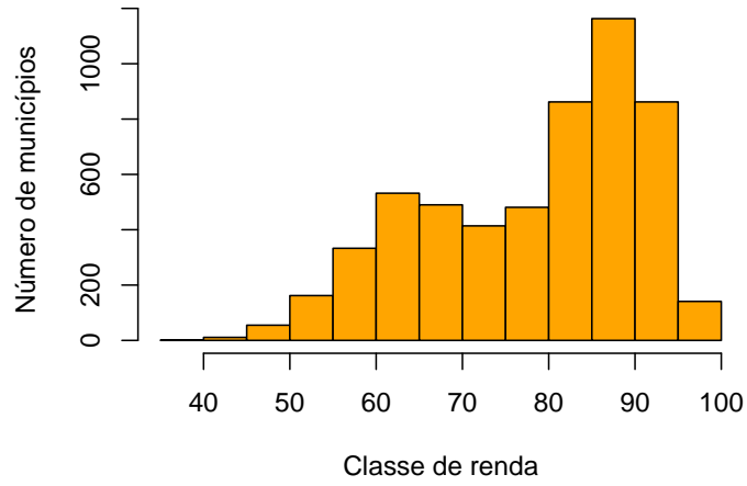
Figura 1: Histograma do alfabetismo.
