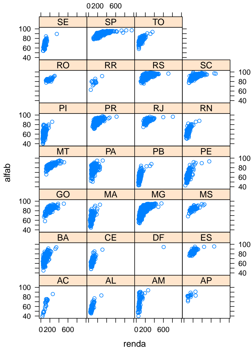
Figura 5: Diagrama de dispersão do alfabetismo em função da renda.
