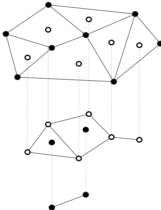
Figura 2.8: Uma subdivisão planar e os seus múltiplos níveis de RAG
