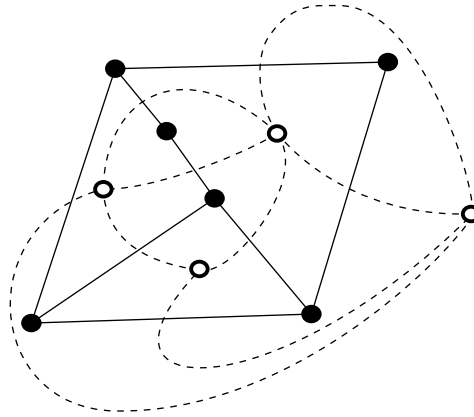
Figura 2.5: Exemplo de uma subdivisão e sua representação dual
