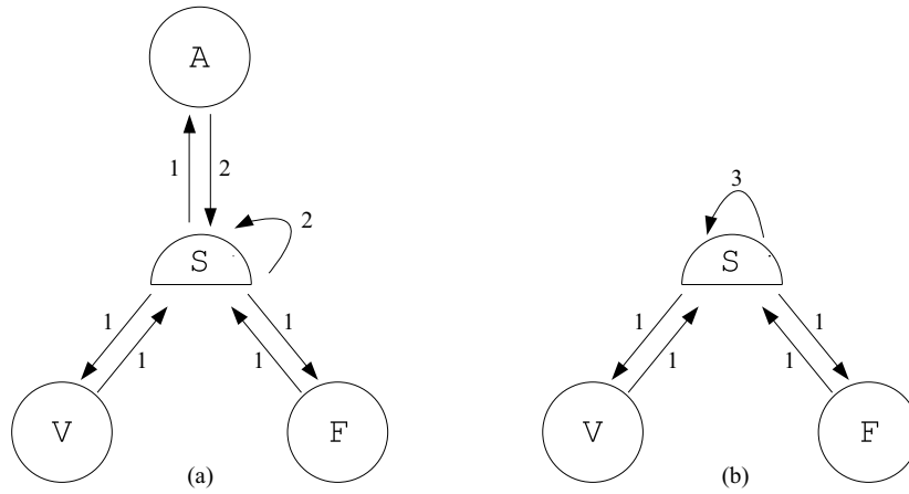
Figura 2.13: Ponteiros das estruturas Half-edge (a) e Vertex(Face)-edge (b)
