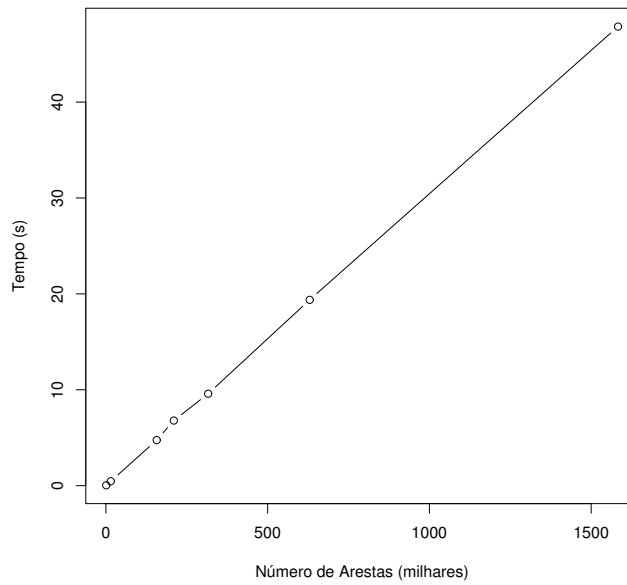
Figura 4.14: Tempos obtidos com a busca de padrões
