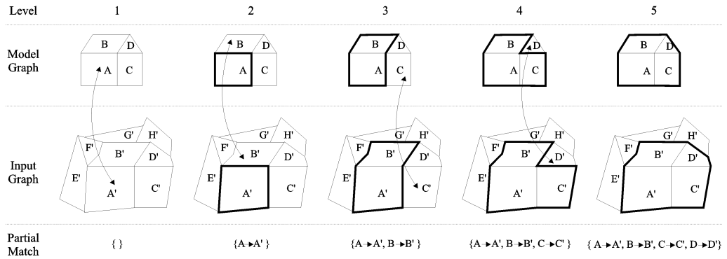
Figura 3.2: Crescimento de regiões [25]
