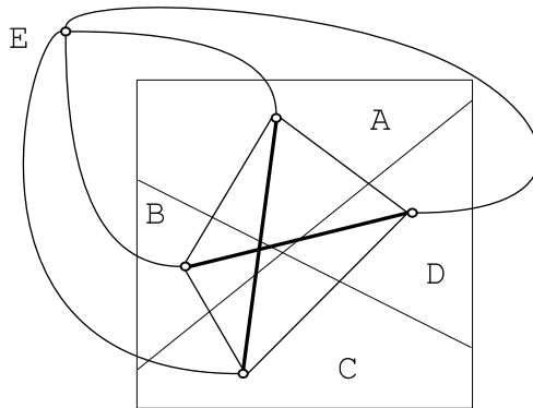
Figura 2.6: Restrições da definição de adjacência para regiões de uma imagem [33]
