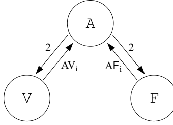
Figura 2.14: Ponteiros da Estrutura de Dados Simétrica
