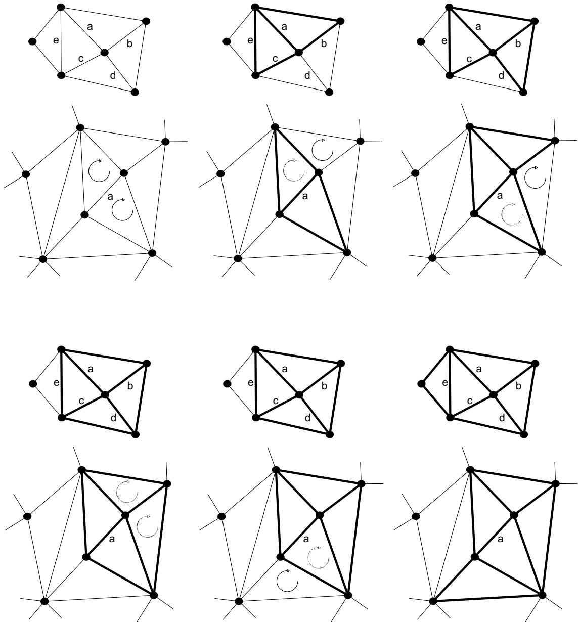
Figura 4.8: Exemplo do algoritmo de isomorfismo
