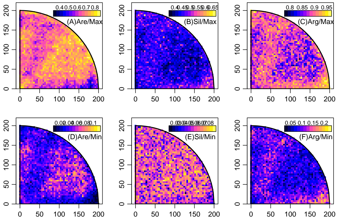
Figura 4.8: Frações máximas e mínimas por componente, obtidas em 1000 simulações para cada localização.
