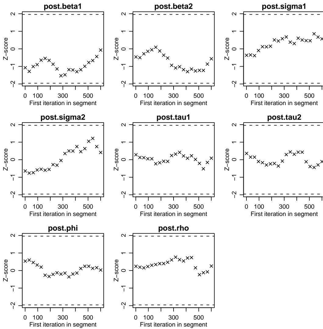
Figura 4.17: Diagnóstico de convergência para o Teste de Geweke. FONTE: A autora (2010).
