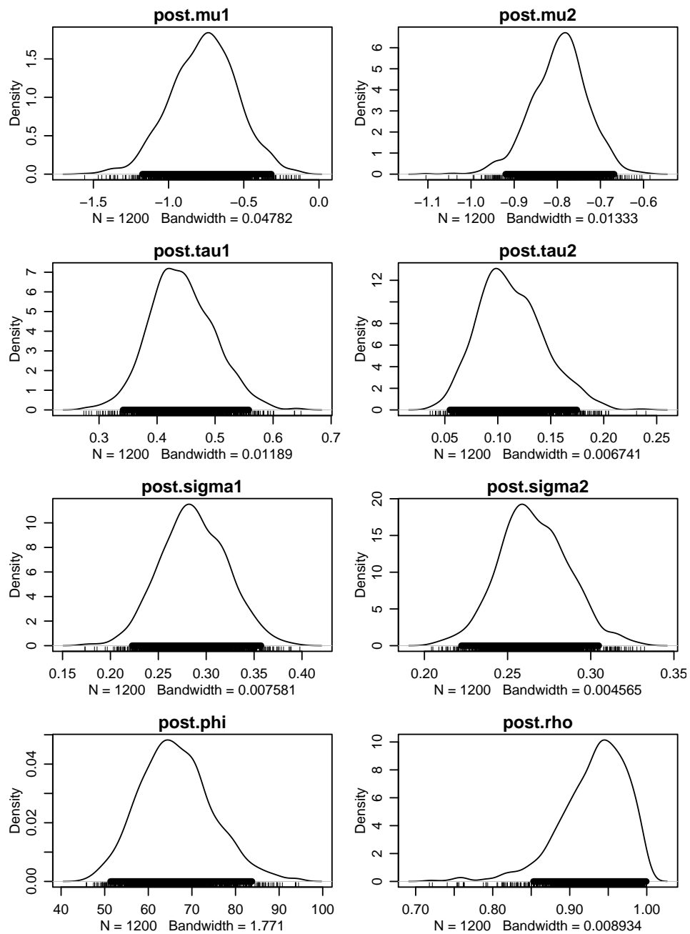
Figura 4.16: Densidades estimadas para as posteriori dos parâmetros com respectivos intervalos de alta densidade a posteriori a 95%. FONTE: A autora (2010).
