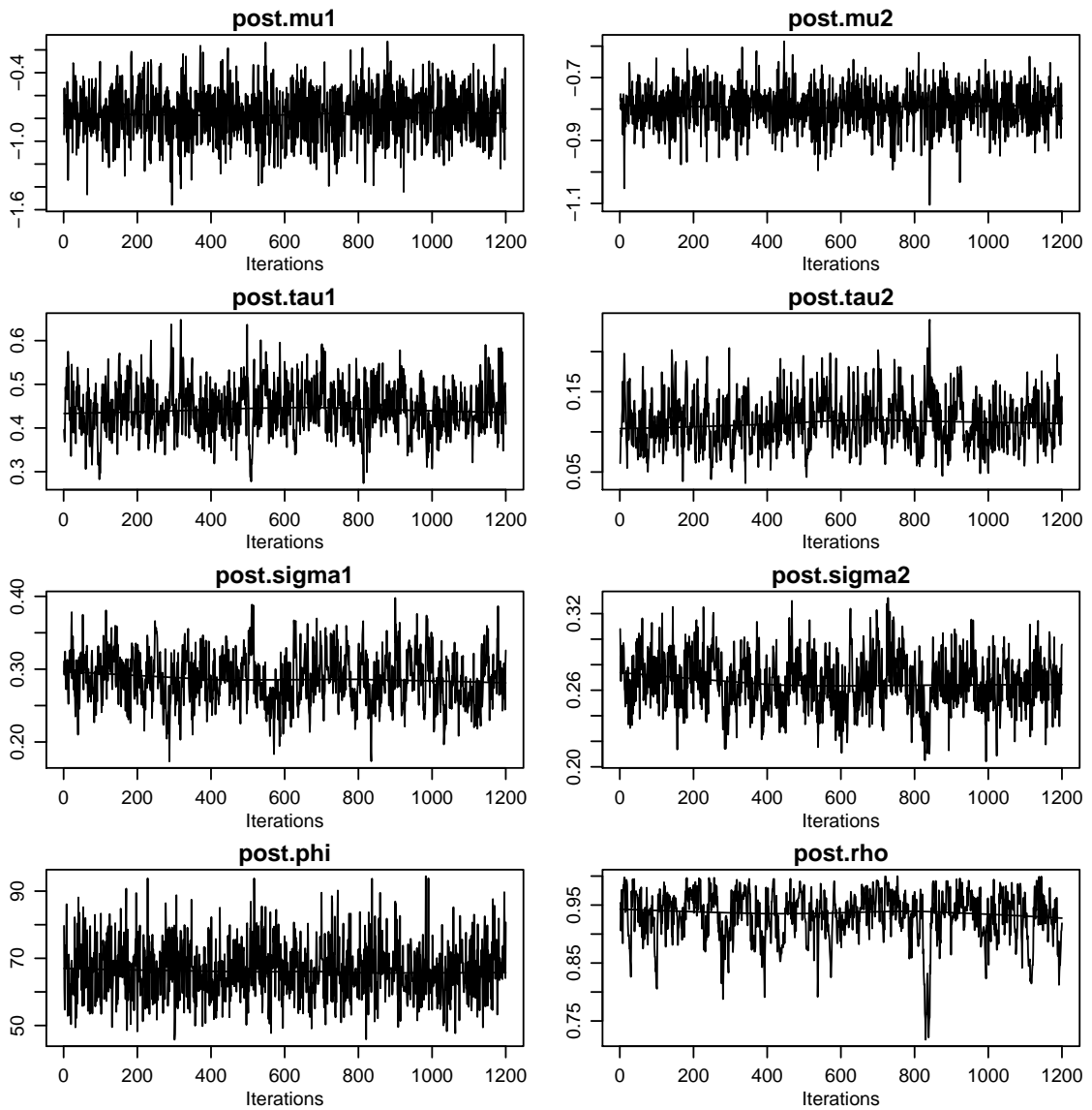
Figura 4.15: Trajetória das posteriori dos parâmetros. FONTE: A autora (2010).
