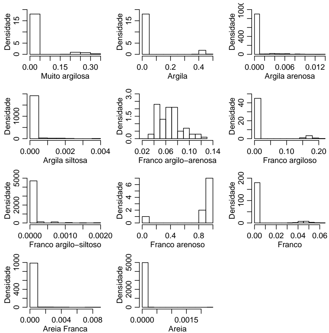
Figura 4.10: Probabilidades a posteriori de classificação nas diferentes classes de solo. FONTE: A autora (2010).
