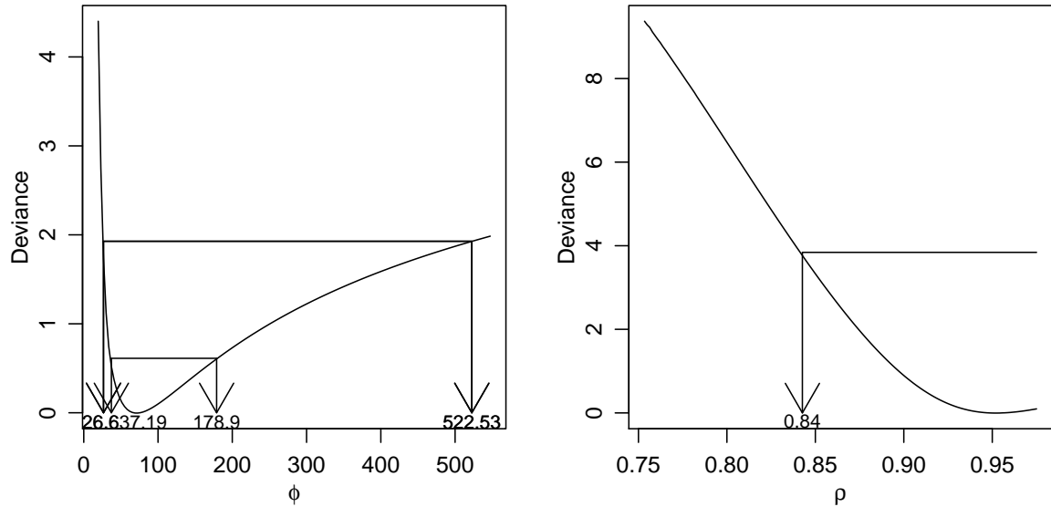
Figura 4.12: Deviance para \phi com linhas de corte de 83,5% e 60% de confiança (esquerda) e para \rho com linhas de corte de 95% de confiança (direita). FONTE: A autora (2010).
