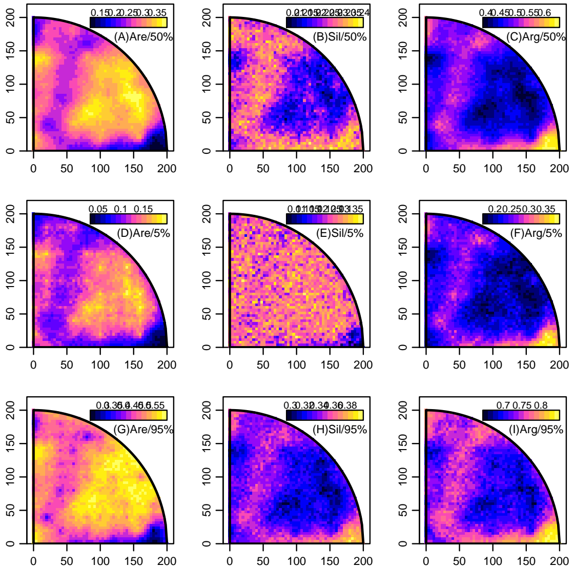
Figura 4.9: Frações medianas, inferiores a 5% e 95% de probabilidade, por componente, obtidos em 1000 simulações para cada localização.
