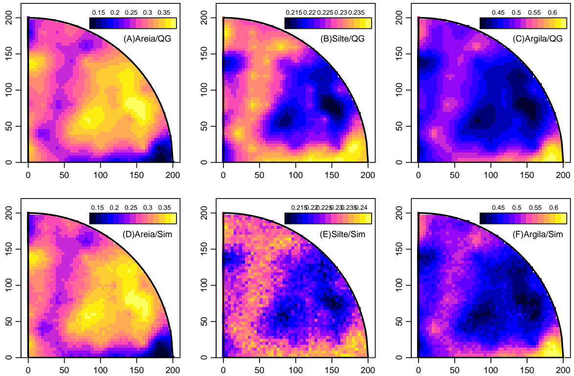
Figura 4.6: Mapas das frações de areia, silte e argila obtidos por quadratura de Gauss-Hermite (A-C) e por simulação (D-F). FONTE: A autora (2010).
