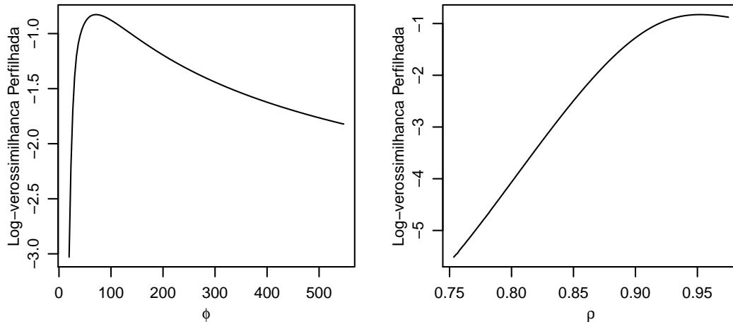
Figura 4.11: Log-verossimilhanças perfilhadas para \phi e \rho . FONTE: A autora (2010).
