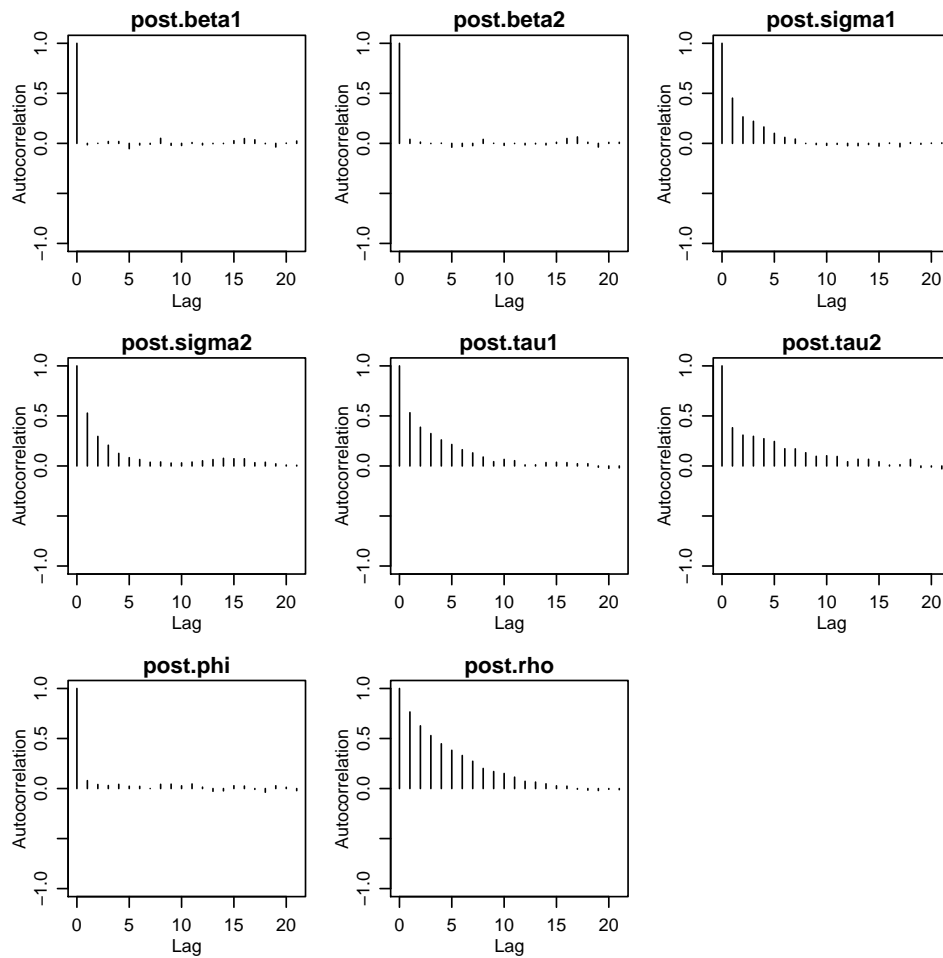
Figura 4.14: Autocorrelações dos parâmetros à posteriori . FONTE: A autora (2010).
