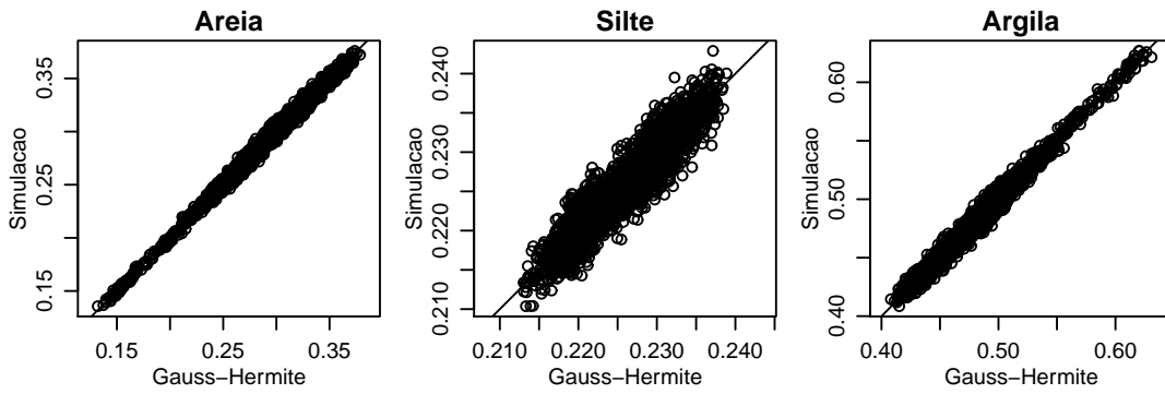
Figura 4.7: Frações de areia, silte e argila obtidos por quadratura de Gauss-Hermite versus simulação.
