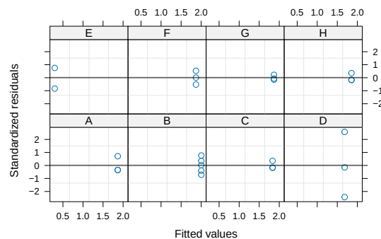
Figura 72: Gráfico de resíduos para cada laboratório do modelo ajustado.
