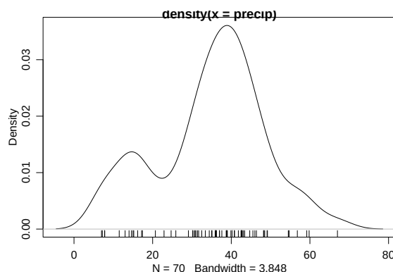
Figura 28: Dados precip e a densidade estimada usando a função density .
