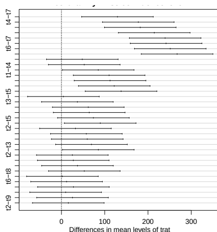
Figura 60: Resultados do teste de Tukey.
