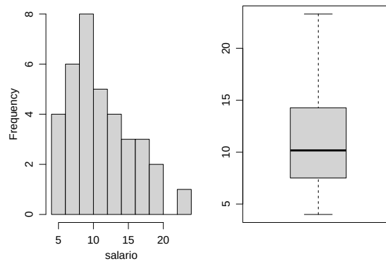
Figura 8: Histograma (esquerda) e boxplot (direita) para a variável salario .
