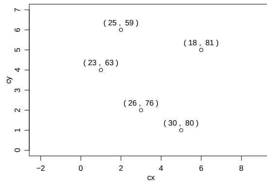
Figura 78: Exemplo hipotético com dois atributos medidos em cinco localizações identificadas por pares de coordenadas. Os valores dos atributos são indicados dentro dos parêntesis.
