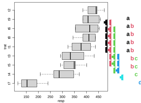
Figura 61: Visualização dos resultados do teste de Tukey com função do pacote multicompView
