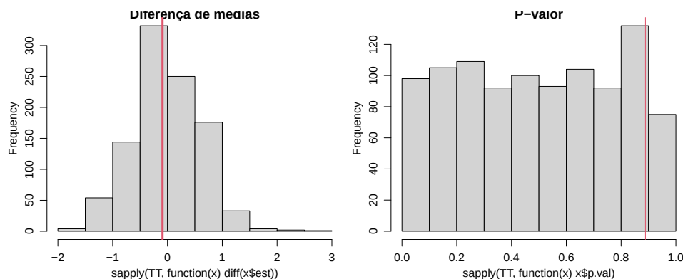
Figura 77: Valores da diferença de médias (esquerda) e p-valor (direita) da amostra (linhas verticais) comparados aos histogramas dos valores obtidos nas reamostras.
