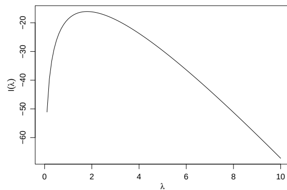
Figura 35: Função de verossimilhança (esquerda) e deviance (direita) para o parâmetro \lambda da distribuição Poisson.
