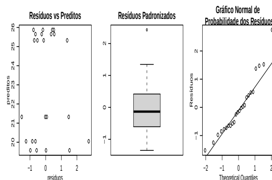
Figura 66: Alguns gráficos de resíduos definidos pelo usuário.
