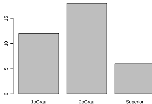
Figura 5: Gráfico de barras para variável instrucao .
