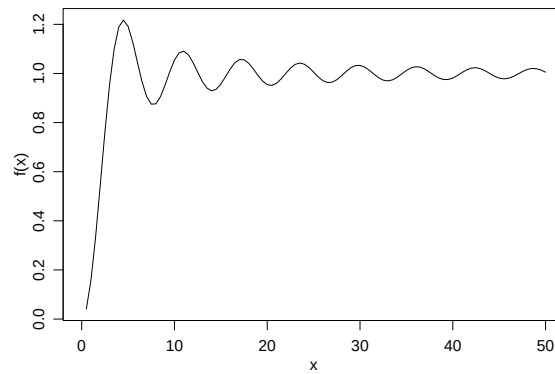
Figura 1: Gráfico da função dada em (a).
