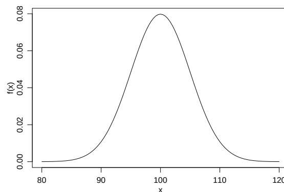
Figura 2: Gráfico da função dada em (b).
