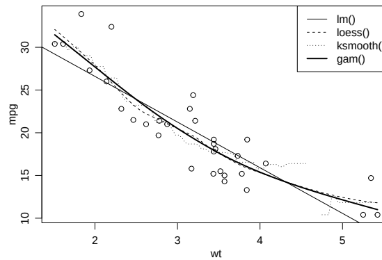
Figura 54: Diferentes modelos ajustados para descrever a relação entre duas variáveis quantitativas.
