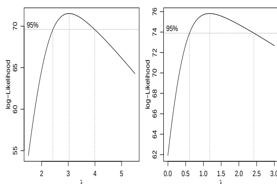
Figura 71: Perfis de verossimilhança do parâmetro da transformação Box-Cox na presença e ausência do ponto atípico do Laboratório E.
