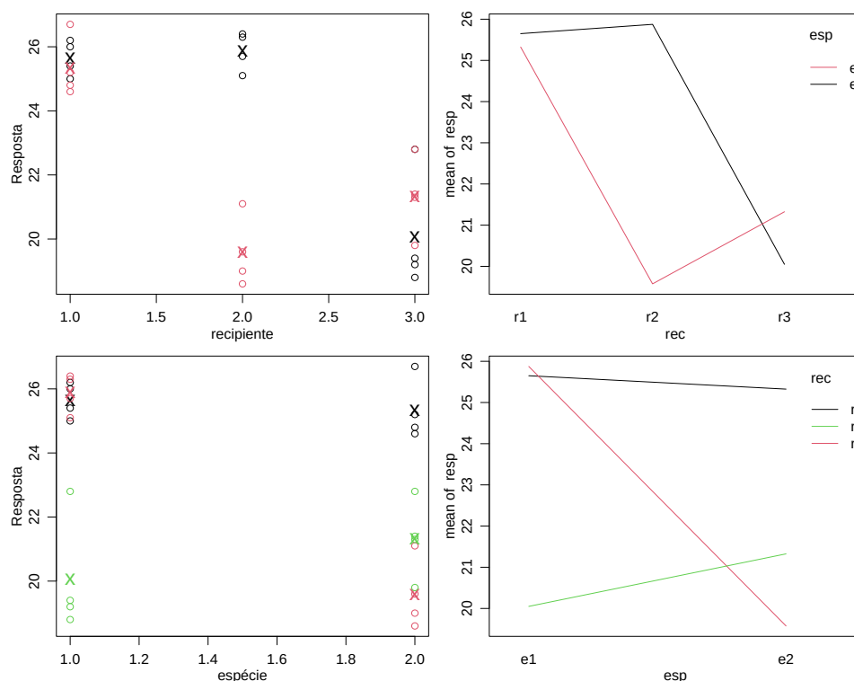
Figura 63: Gráficos de pontos examinando a interação entre os fatores.
