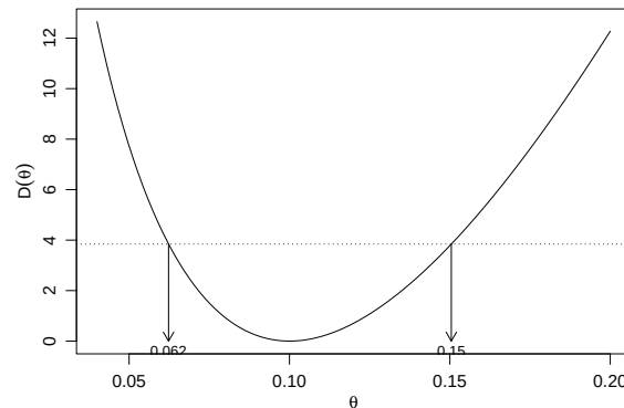
Figura 43: Obtenção gráfica do IC para o parâmetro \theta da \text{Exp}(\theta) para uma amostra de tamanho 20 e média 10.
