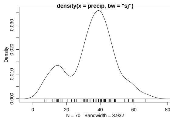
Figura 32: Densidade estimada para os dados precip usando a função density com critério de Sheather & Jones para seleção da largura de banda.
