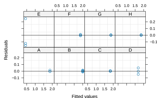
Figura 70: Gráfico de resíduos para cada laboratório do modelo ajustado.
