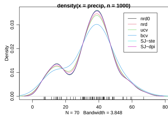
Figura 33: Diferentes métodos para largura de banda implementados pela função density .
