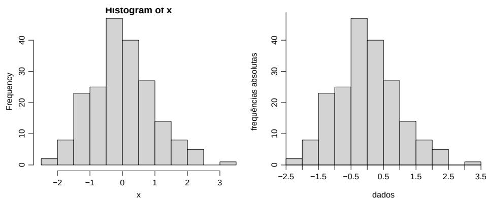
Figura 12: Histograma gerado com opções padrão (esquerda) e modificadas (direita).
