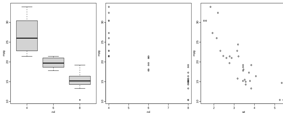
Figura 52: Exemplos de gráficos definidos através de fórmulas.
