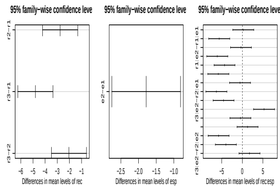
Figura 67: Visualização dos resultados do teste de Tukey de comparações múltiplas.
