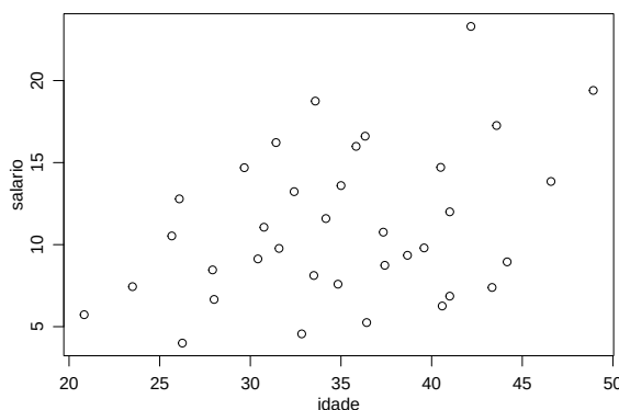
Figura 11: Diagrama de dispersão para as variáveis salario e idade .
