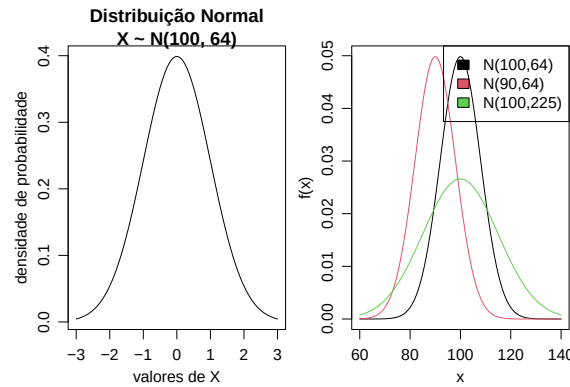
Figura 22: Gráfico com texto nos eixos e título (esquerda) e várias distribuições em um mesmo gráfico (direita).
