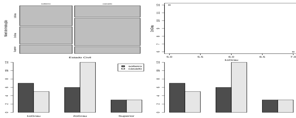
Figura 14: Representações gráficas de tabelas de contingência de duas variáveis obtidas pelas funções table() e fable() .
