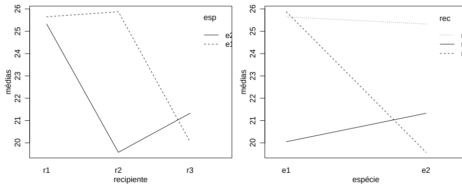
Figura 62: Gráficos de interação entre os fatores.
