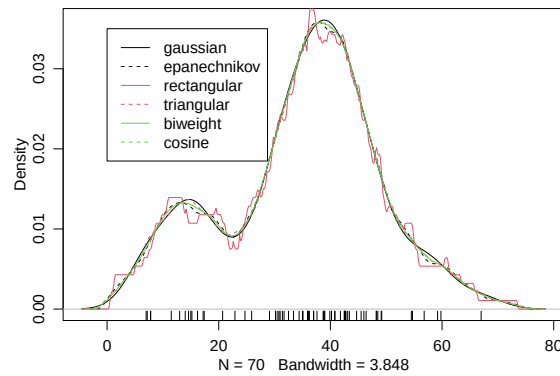
Figura 31: Densidade estimada usando a função density com diferentes valores para o argumento kernel .
