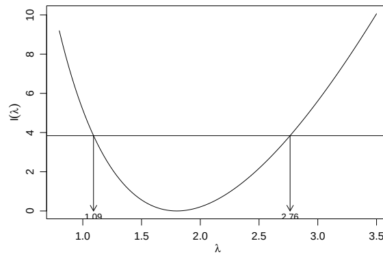
Figura 36: Intervalo de confiança baseado na deviance para o parâmetro \lambda da distribuição Poisson.
