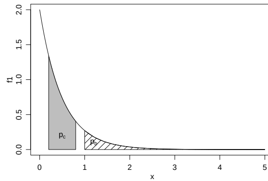
Figura 17: Probabilidades pedidas nos itens (b) e (c) do Exemplo 1.
