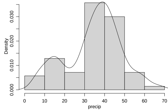
Figura 27: Histograma para os dados precip e a densidade estimada usando a função density .
