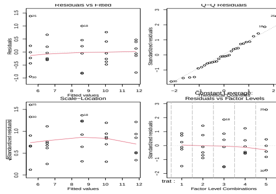
Figura 50: Gráficos de diagnóstico para dados transformados
