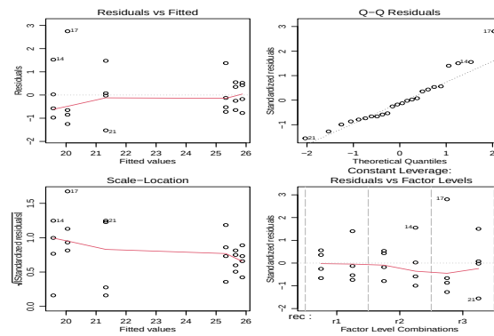
Figura 64: Gráficos de resíduos produzidos para objetos da classe lm .
