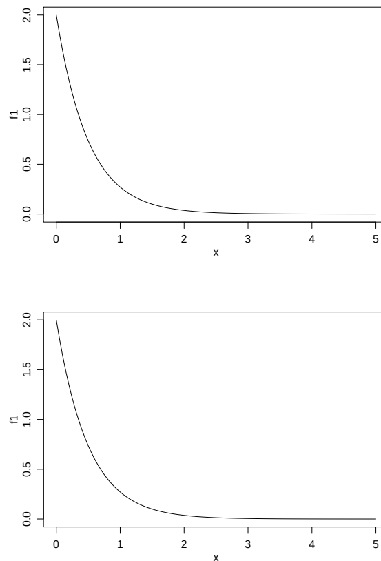
Figura 16: Gráfico da função de probabilidade do Exemplo 1.
