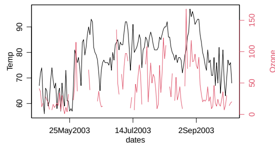
Figura 13: Ilustração de gráfico com duas escalas para o eixo- y : evolução dos valores de temperatura e ozônio.
