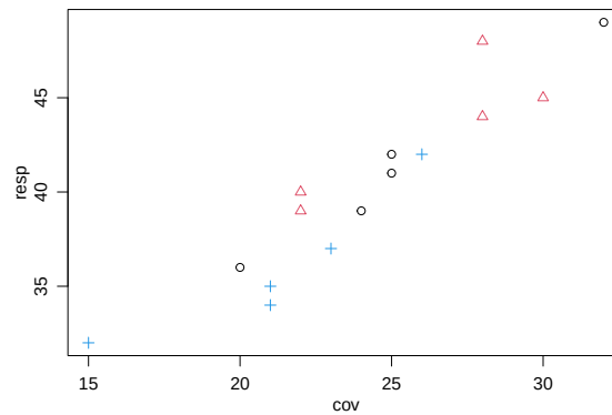
Figura 68: Dados para análise de covariância.
