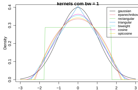
Figura 30: Diferentes núcleos implementados pela função density .
