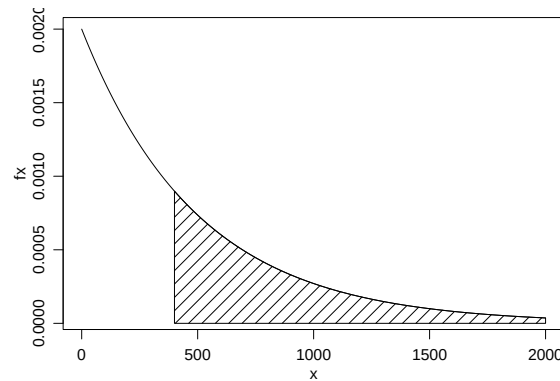
Figura 25: Função de densidade da Exp(500) com a área correspondente à P[X \geq 400] .
