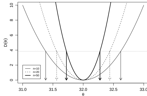
Figura 41: Funções deviance para o parâmetro \theta da N(\theta, 1) para amostras de média 32 e tamanhos de amostra n = 10, 20 e 50 .
