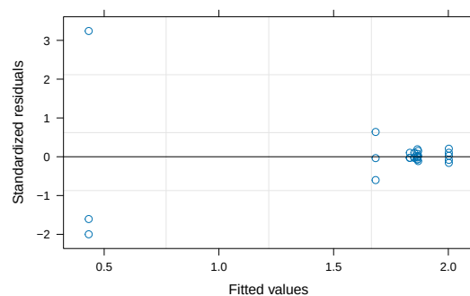
Figura 69: Gráfico de resíduos do modelo ajustado
