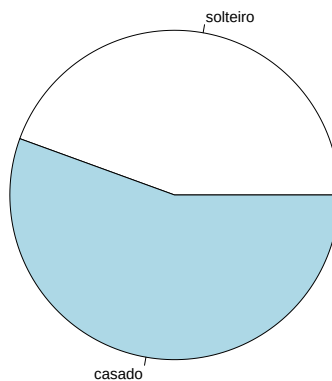
Figura 4: Gráfico de setores para variável civil .
