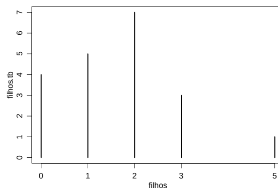
Figura 6: Gráfico de frequências absolutas para variável filhos .
