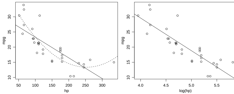
Figura 55: Ilustração do uso de operadores aritméticos e funções polinomiais na especificação de fórmulas.
