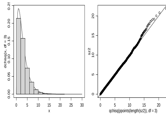
Figura 75: Histograma da uma amostra da soma dos quadrados de três valores da normal padrão e a curva teórica da distribuição de \chi^2_{(3)} (esquerda) e o respectivo qq-plot .
