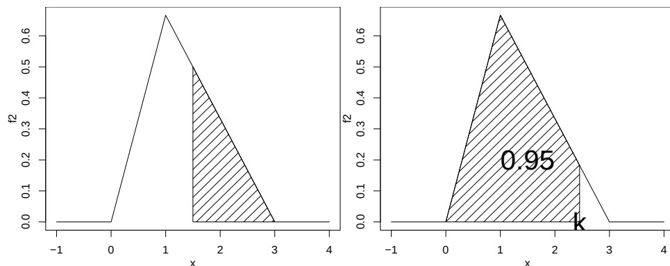
Figura 19: Gráficos indicando as soluções dos itens (a) e (c) do Exemplo 2.
