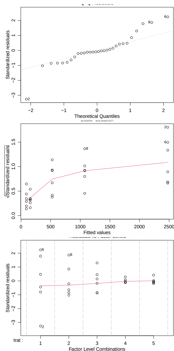
Figura 48: Gráficos de diagnóstico para dados originais
