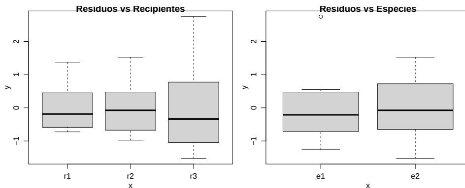
Figura 65: Gráficos de resíduos para cada um dos fatores.
