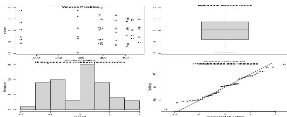
Figura 59: Gráficos de resíduos.
