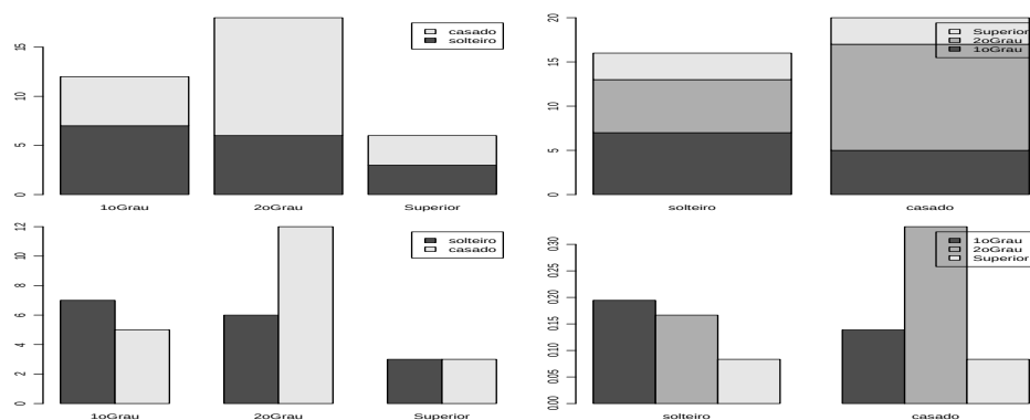
Figura 9: Quatro tipos de gráficos de barras ilustrando o resultado do cruzamento das variáveis civil e instrucao.
