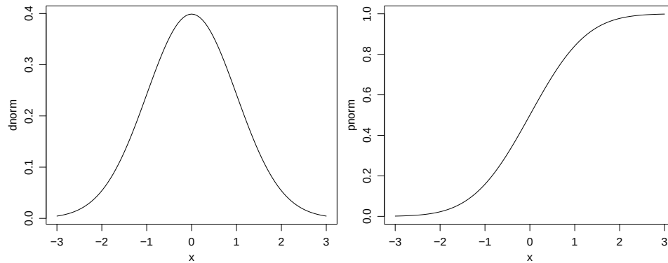
Figura 20: Funções de densidade e probabilidade da distribuição normal padrão.
