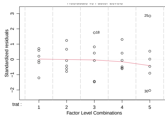
Figura 51: Gráficos de diagnóstico para dados com transformação logarítmica
