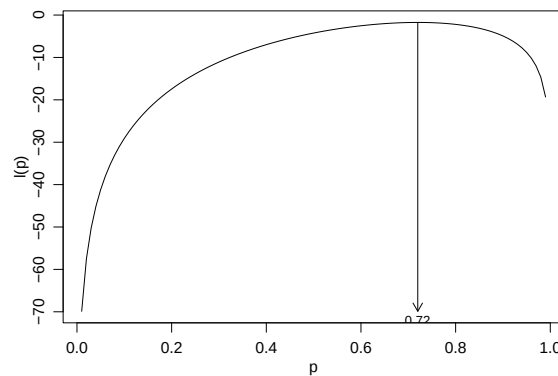
Figura 38: Função de verossimilhança para o parâmetro p da distribuição Bernoulli.
