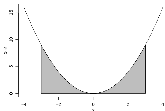
Figura 3: Gráfico onde a área indicada corresponde à integral definida na equação 2.
